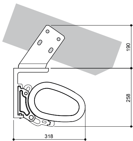
Dachsparrenmontage
