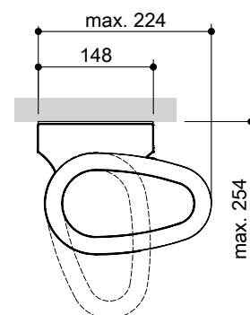
bei Deckenmontage 5°-80° CLEO 5530
