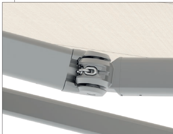
Gelenkarm mit Kette
