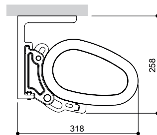
Deckenmontage
