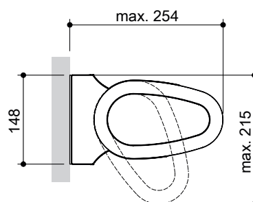
bei Wandmontage 5°-65° CLEO 5530
